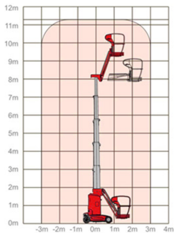
Arbeitsdiagramm Reichweite
