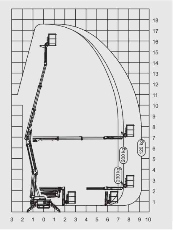
Arbeitsdiagramm Reichweite
