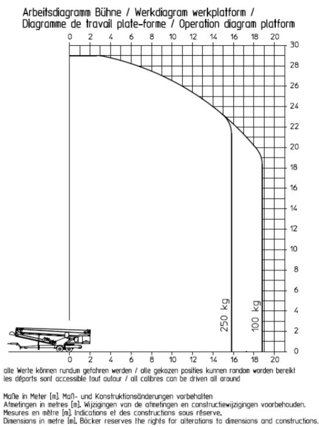
Arbeitsdiagramm Reichweite
