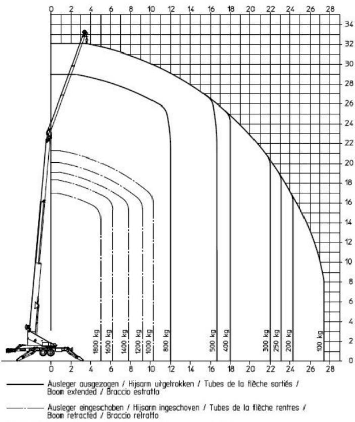
Arbeitsdiagramm Reichweite
