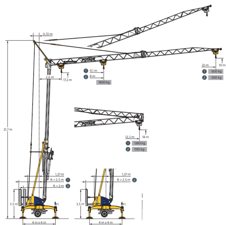
Arbeitsdiagramm Reichweite
