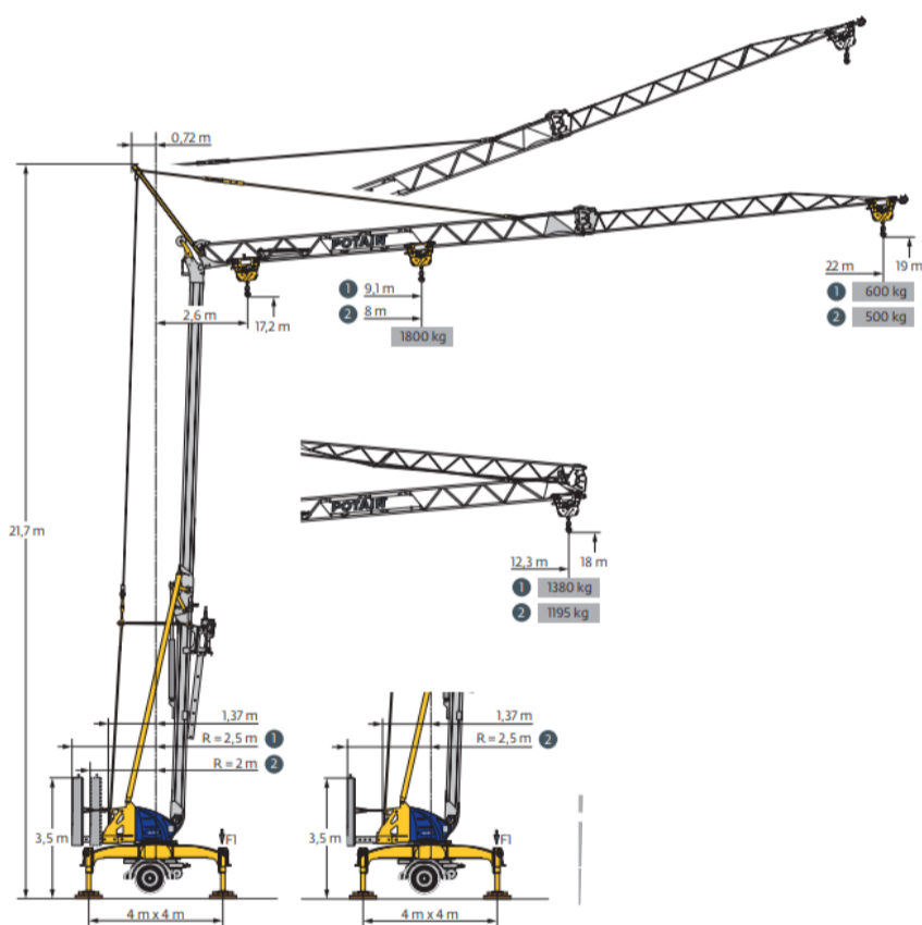
Arbeitsdiagramm Reichweite
