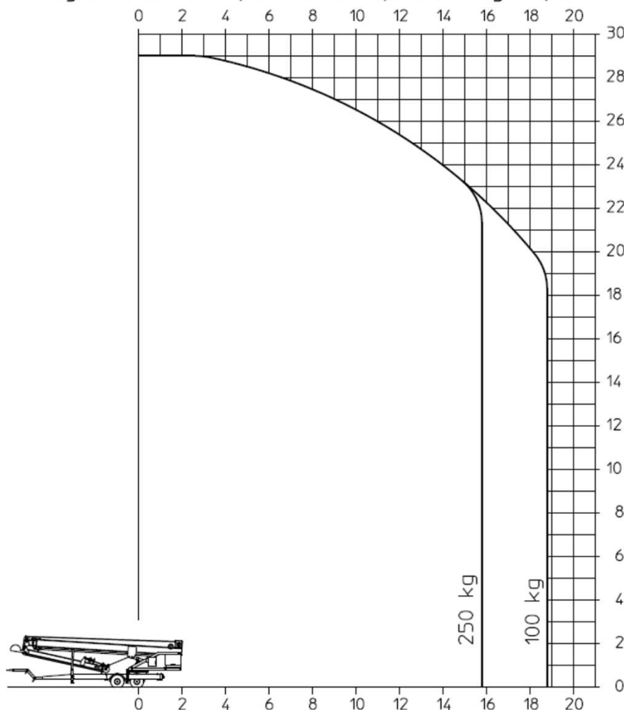
Arbeitsdiagramm Bühne / Werkdiagramm werkplatform / Diagramme de travail plate-forme / Operation diagram platform
